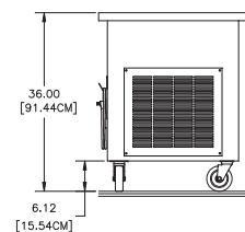
TYP END VIEW
