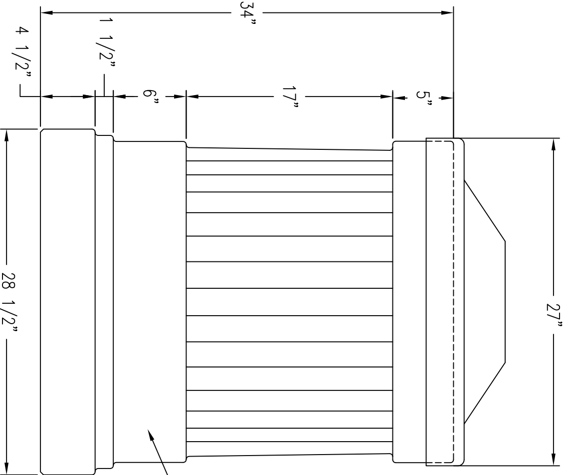
1 ELEVATION VIEW Scale: 1/8" = 1"
