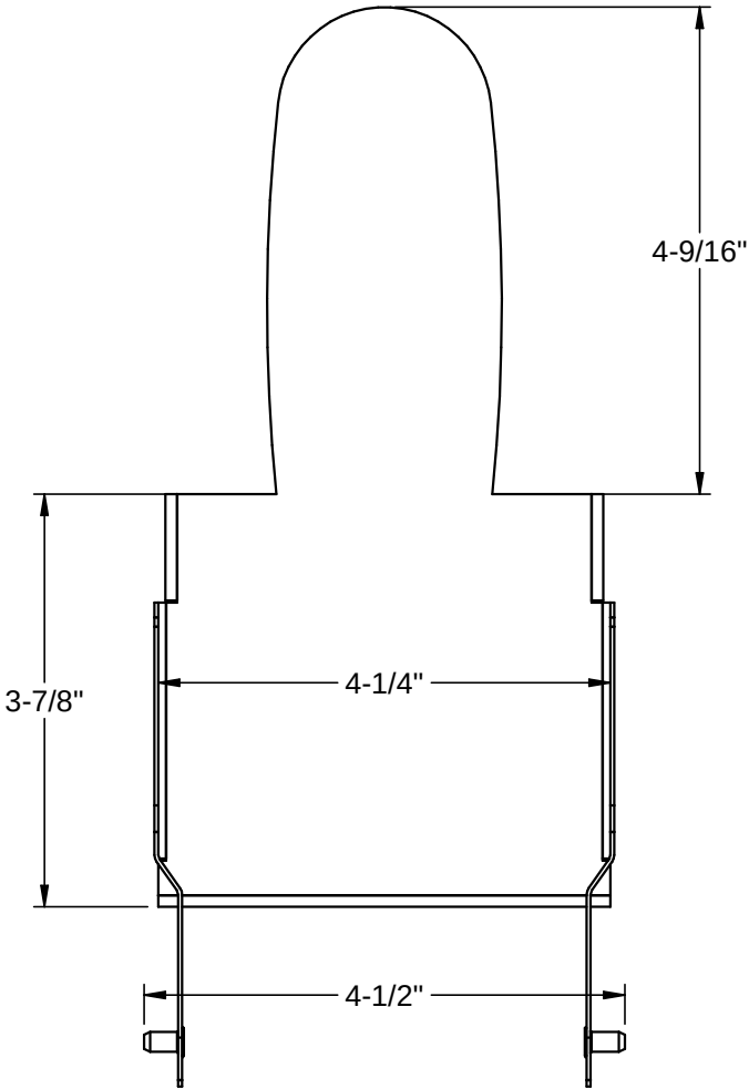
PLAN SCALE: 6" = 1'-0"
