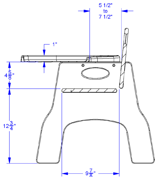
SECTION A-A
