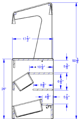
SECTION A-A
