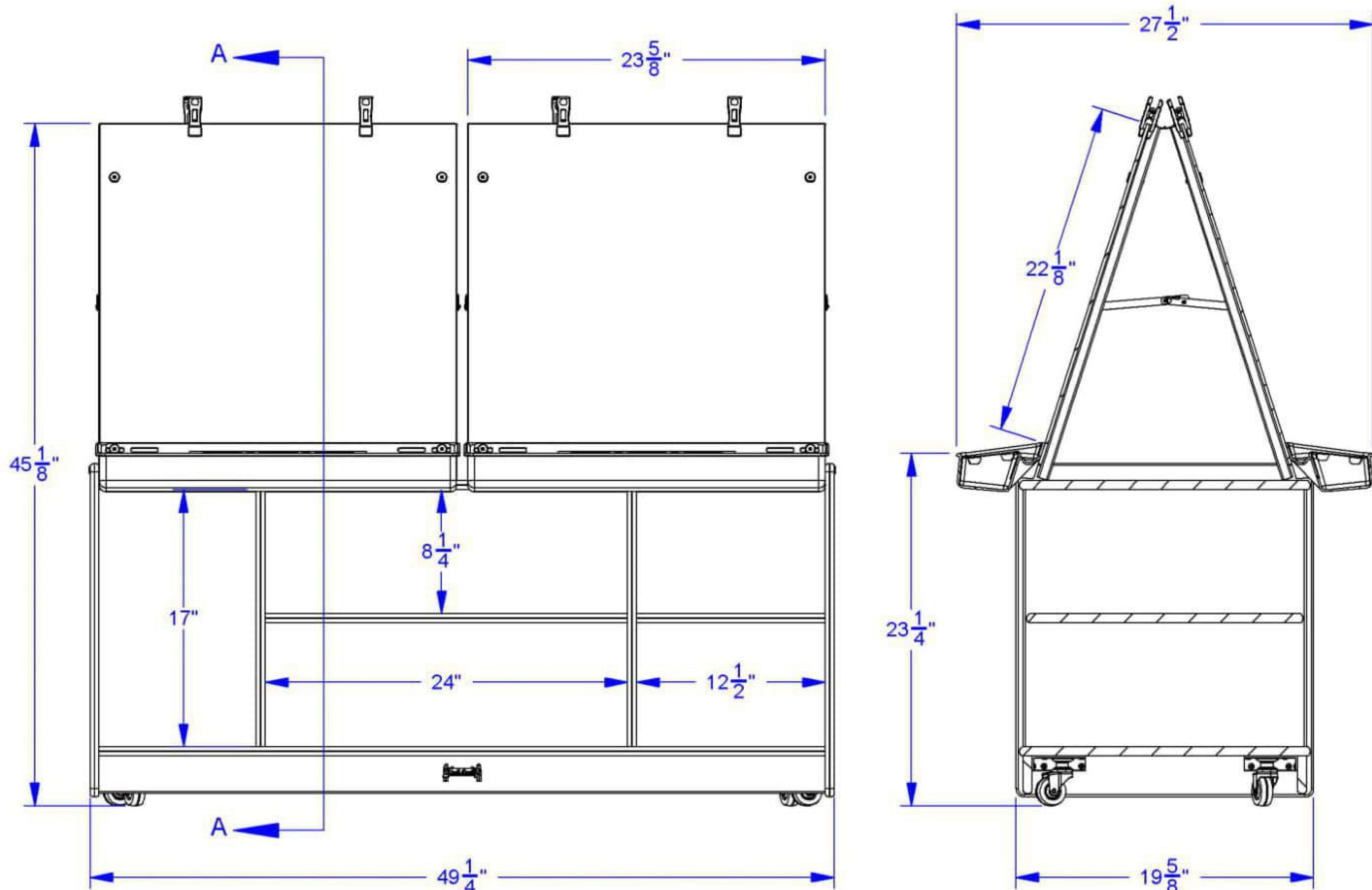
SECTION A-A
