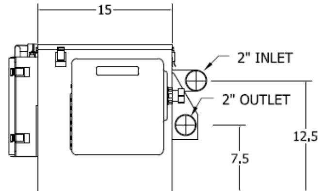
END ELEVATION
