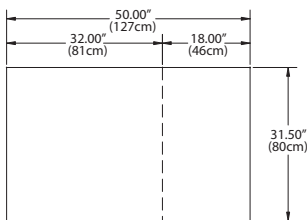
Plan View 18650VDR, 18650VDR-CE
