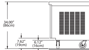
Right End View 18650VDR, 18650VDR-CE, 18682VDR, 18682VDR-CE
