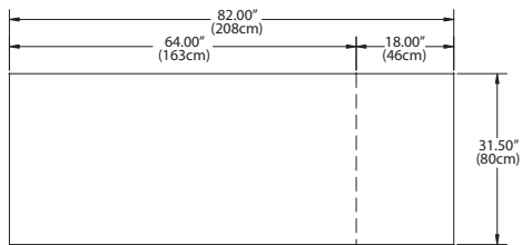
Plan View 18682VDR, 18682VDR-CE
