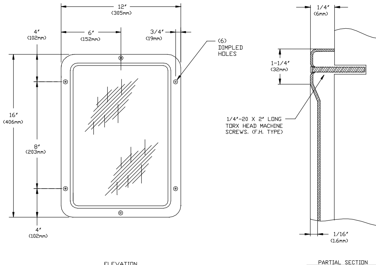
ELEVATION
