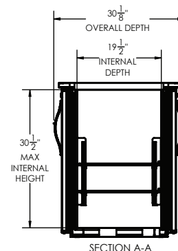
SECTION A-A
