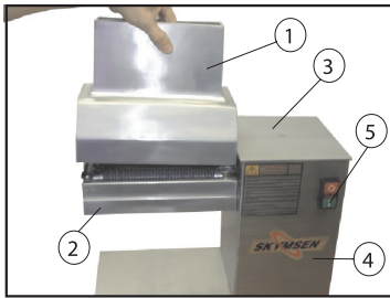
1. Protection lid
