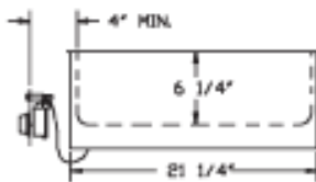
CUTOUT DIMENSIONS
