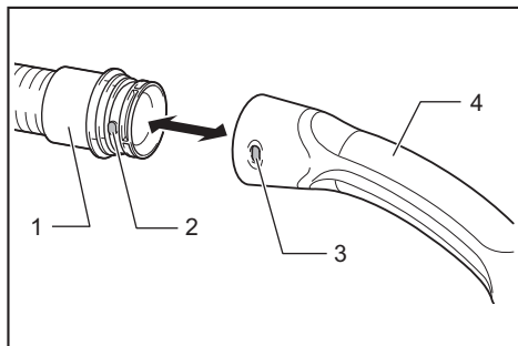
► 1. Extremo de manguera 2. Lengüeta 3. Orificio 4. Conjunto de tubo curvo
