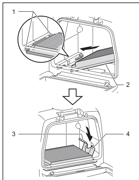
► 1. Soporte 2. Filtro HEPA 3. Varilla 4. Lengüeta
