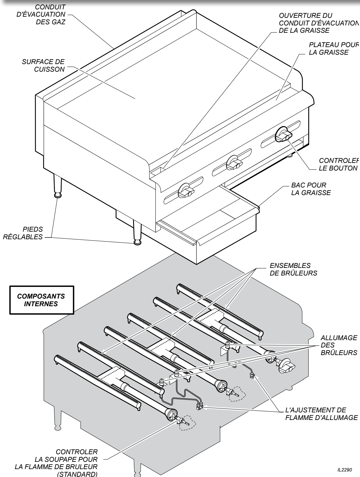
Fig. 5 FONCTIONNALITÉS ET COMMANDES DU GRILL PROFESSIONNEL À GAZ
