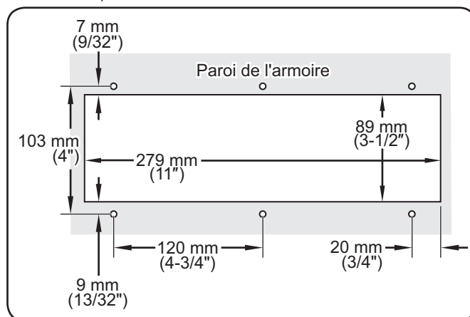
Dimensions des emplacements d'orifices de passage de vis et de découpe pour le panneau de commande
