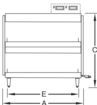
GRSDH—Rayonnage Double
