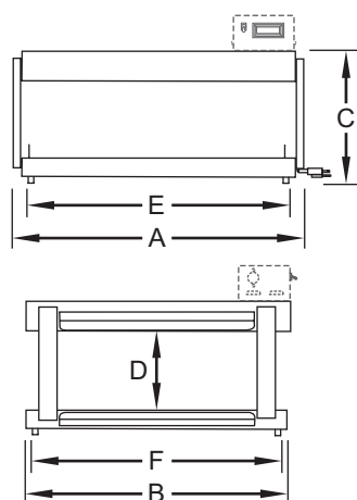
GRSDH—Rayonnage Simple
