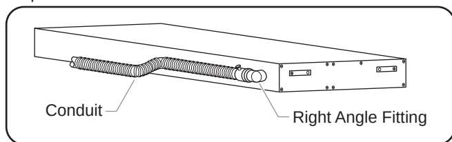
Conduit Connections
