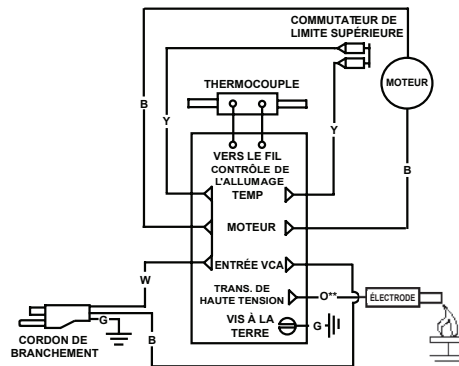
DIAGRAMME DE CONNEXION
