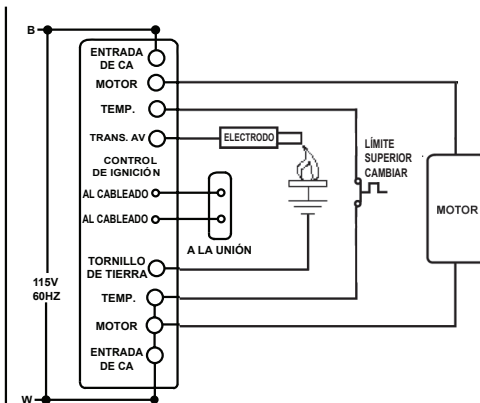
DIAGRAMA ESQUEMÁTICO
