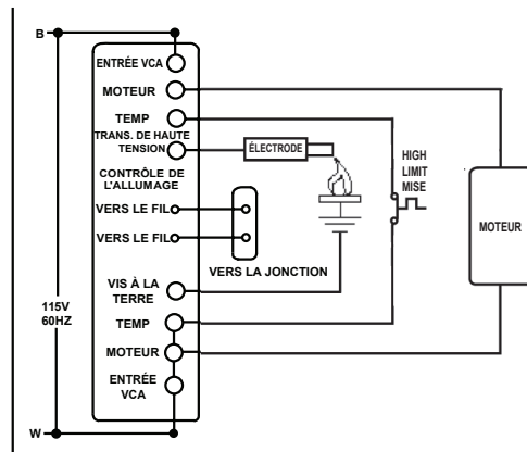
DIAGRAMME SCHÉMATIQUE
