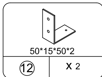
ANGLE BRACKET Escuadra ÉQUERRE TJH3506
