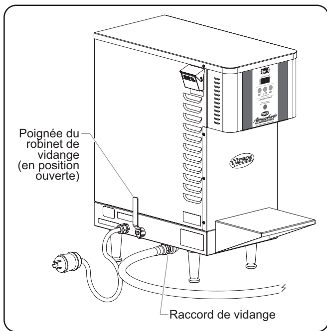
Vidange d'eau
