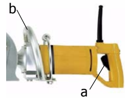
Abbildung 2: Schalterbetätigung
