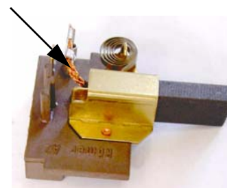
Abbildung 9: Schleifkohle
