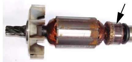
Abbildung 10: Anker
