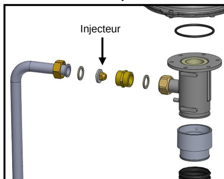
Position injecteur
