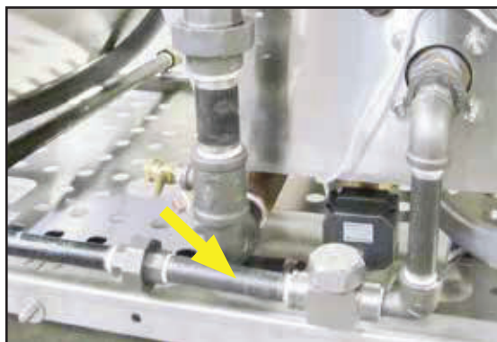
Fig. 11 - Condensate return.
