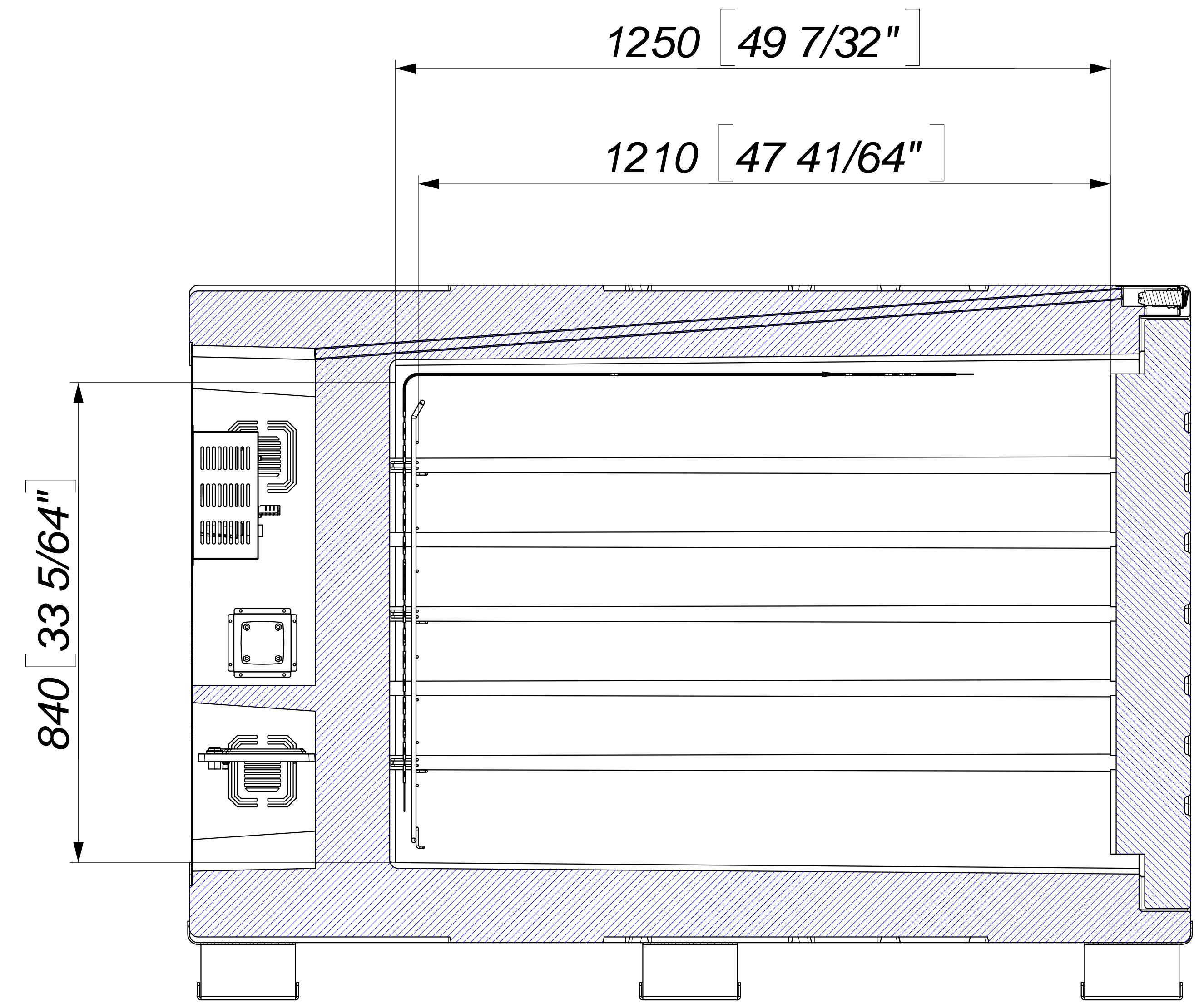
Sezione E-E SCALE 1 : 6
