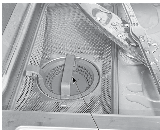
CANASTO COLADOR EN POSICIÓN DE BLOQUEO
