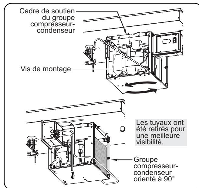
Rotation du groupe compresseur-condenseur
