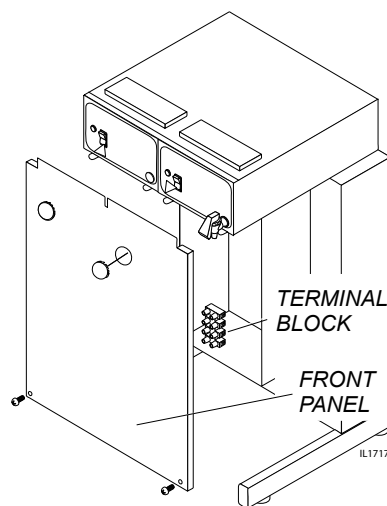
Fig. 3 115/230 Volt Terminal Block
