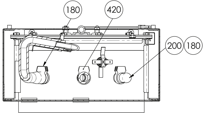
SECTION B-B SCALE 1 : 2
