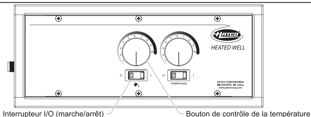
Boutier de commande HWBI-2DA (unité avec orifice de vidange et fonction d'auto-remplissage)
