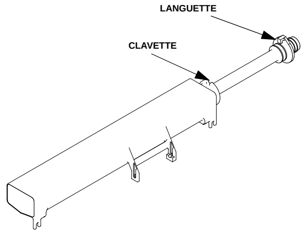
Démontage du tube de distribution d'eau Q130
