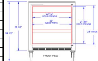
UCR/UCF27 FRONT
