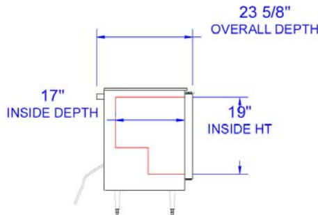
UCR34 FRONT
