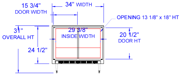
UCR34 FRONT
