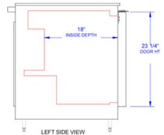
UCR/UCF27 END
