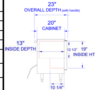
UCR/UCF20 END
