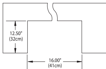
Cutout Dimensions
